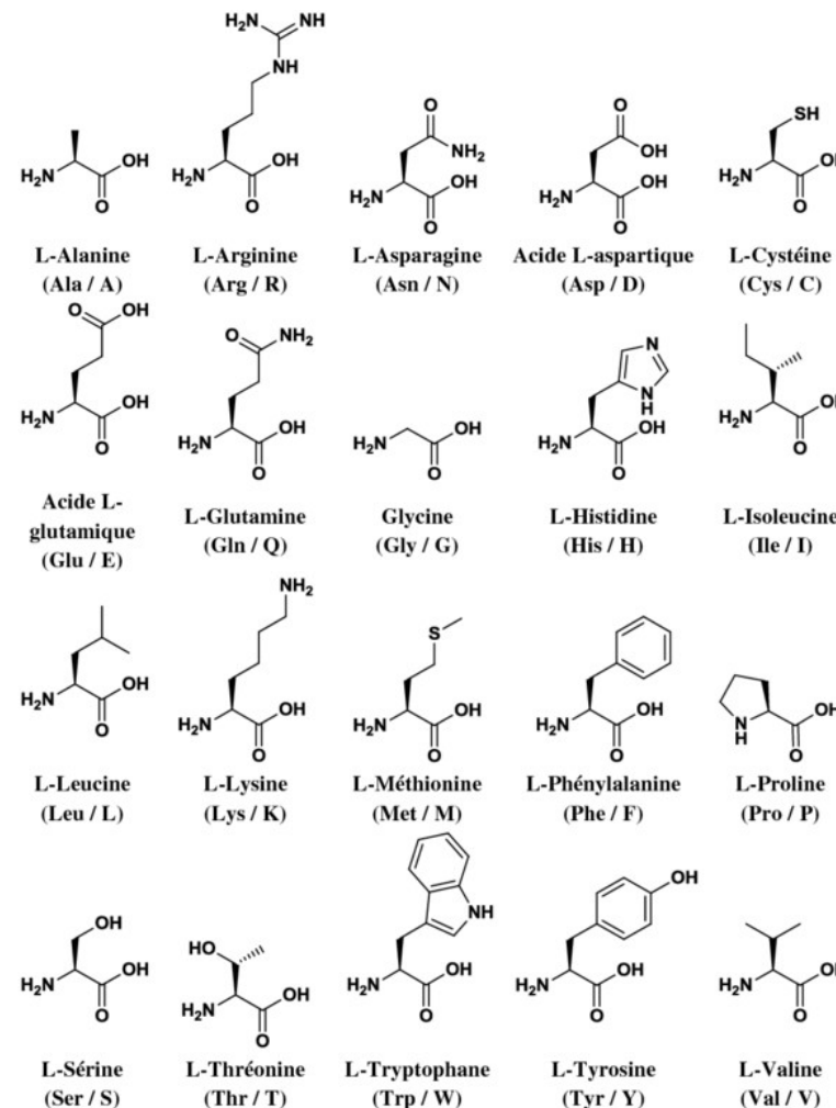
Figure 1. Les 20 acides \alpha -aminés naturels accompagnés de leur code à trois lettres et de leur code à une lettre.
