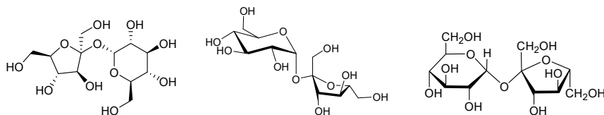
Figure 10. Différentes représentations du saccharose.
